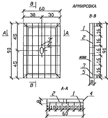
ДЕТАЙЛ НА КАПАК ЗА ШАХТА 60/90
