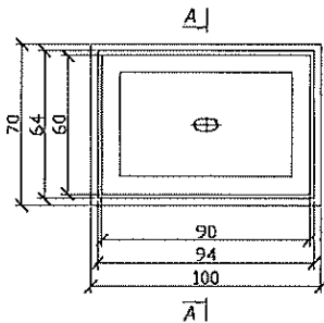
ДЕТАЙЛ - ШАХТА 60/90
