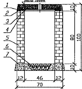
РАЗРЕЗ А-А
